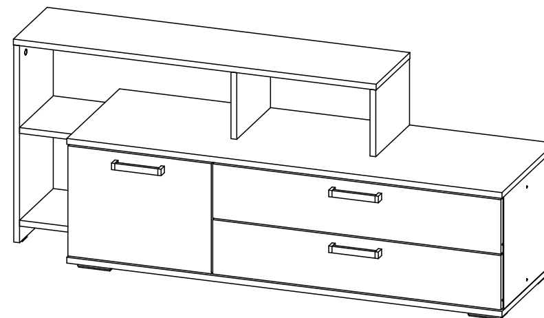
«Санса» ТВ 01 Тумба под ТВ ↔ 1400 ↑ 565 ↗ 400 «Sansa» TB 01 TV cabinet
