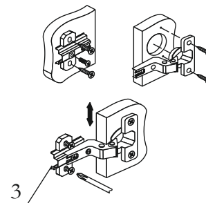
Регулировка створки по высоте
