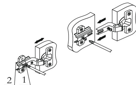
Регулировка створки по ширине
